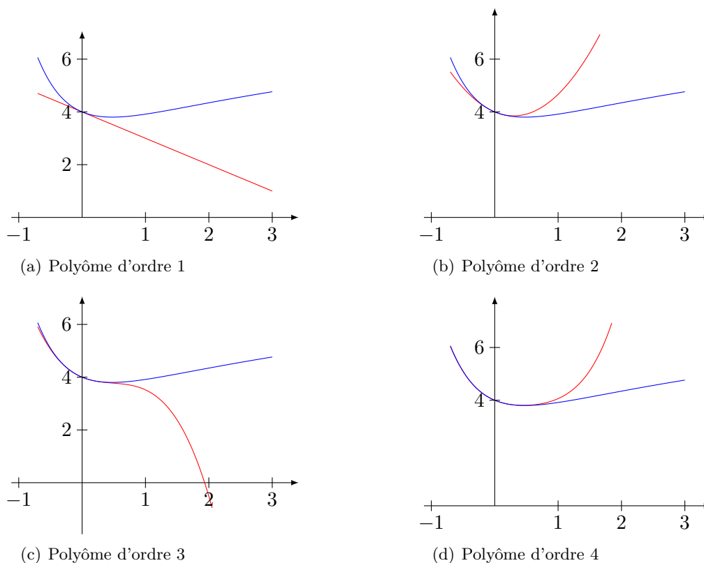
FIGURE 12.12 – Les développements limités d'ordre de plus en plus grand de la fonction de l'exemple 12.475. La fonction est en bleu et les « approximations » sont en rouge.
