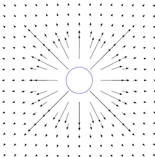
FIGURE 12.13 – Le champ de gravitation de la Terre.
