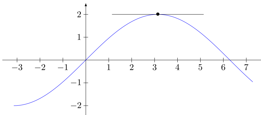
FIGURE 12.9 – Tangentes au graphe d'une fonction d'une variable
