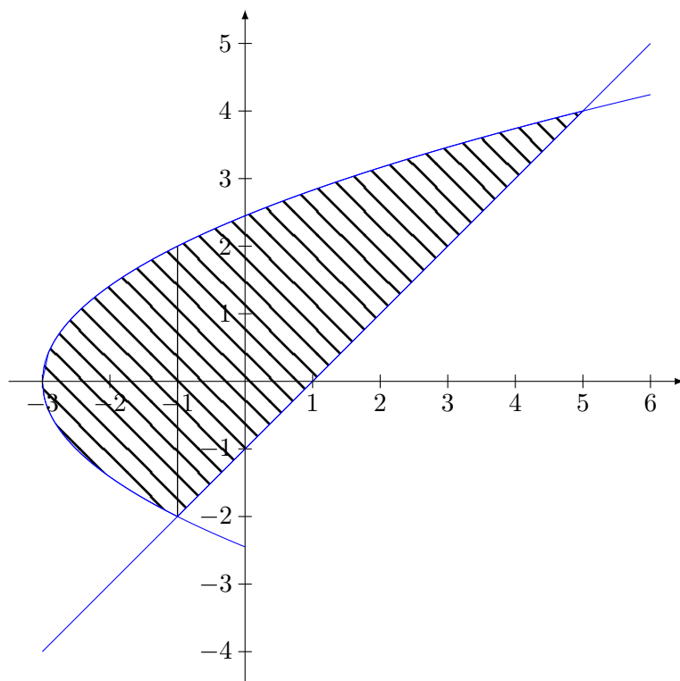
FIGURE 20.19 – La région D de l'exemple 20.193
