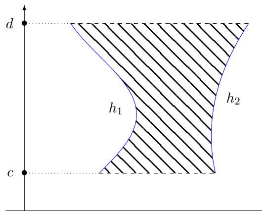
(b) Une région du deuxième type
