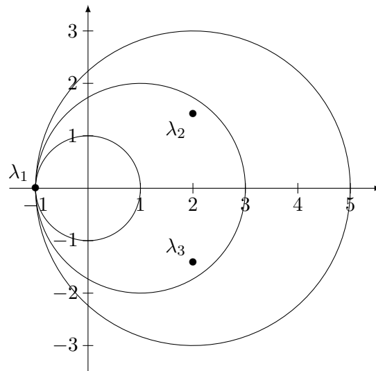
FIGURE 36.2 – Les disques de Gershgorin et les valeurs propres pour l'exemple 36.156.
