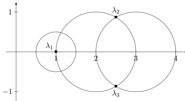
FIGURE 36.1 – Les disques de Gershgorin et les valeurs propres pour l'exemple 36.155.
