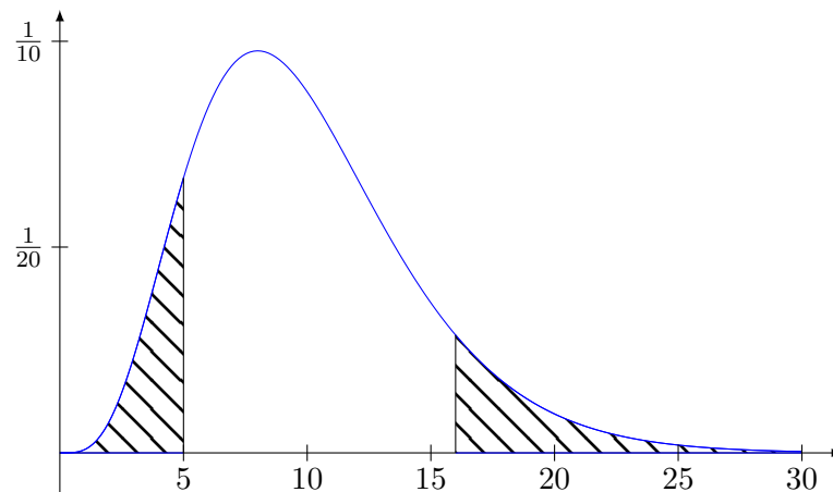
FIGURE 39.3 – L'intervalle de confiance pour une \chi^2 .
