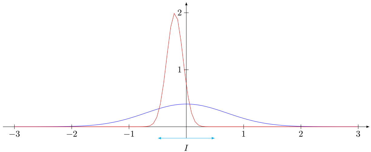
FIGURE 39.1 – Un estimateur sans biais et un avec biais.
