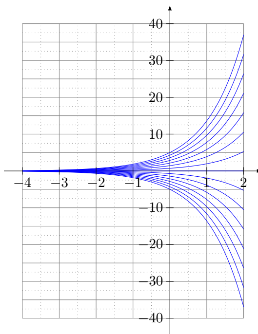
FIGURE 34.1 – Quelques trajectoires de l'équation y' = y .
