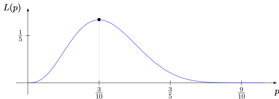
FIGURE 39.2 – La fonction de vraisemblance de l'exemple 39.28.
