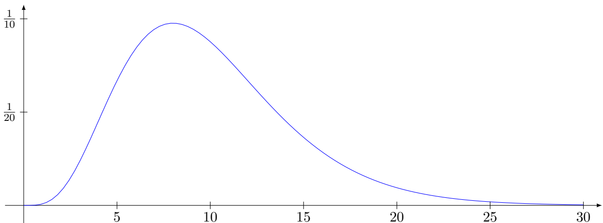
FIGURE 38.1 – La densité de \chi^2(10) .
